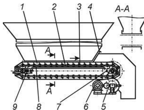
Рис. 1 Схема пластинчастого живильнику
