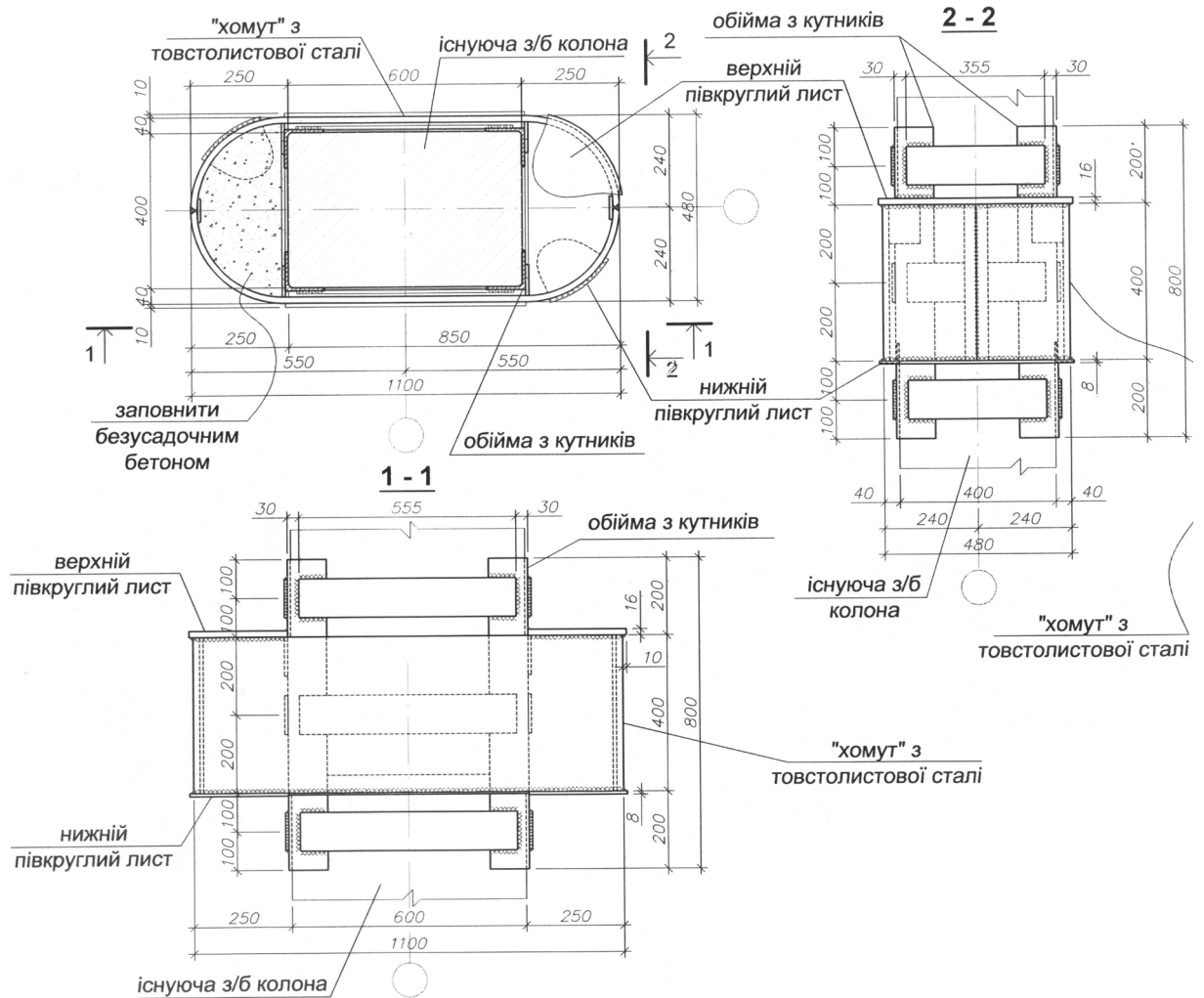
Рис. 3. Нова конструкція метало-бетонної консолі
