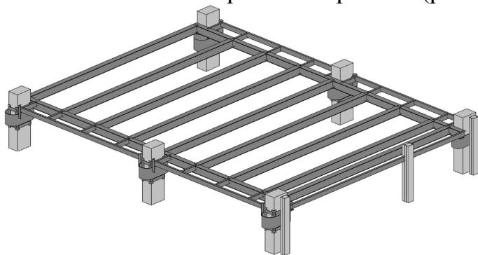
Рис. 4. Конструкція балочного перекриття із спиранням на метало-бетонні консолі
